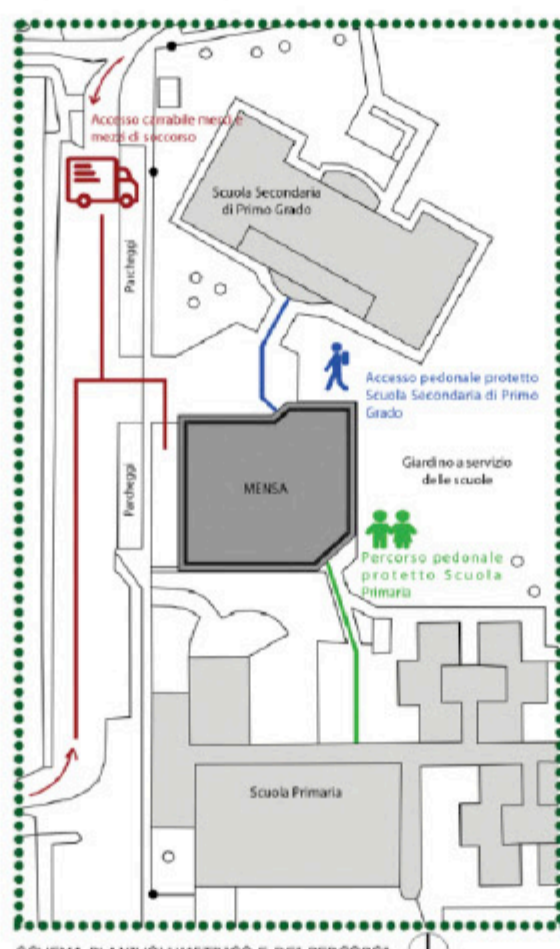
SCHEMA PLANIVOLUMETRICO E DEI PERCORSI
